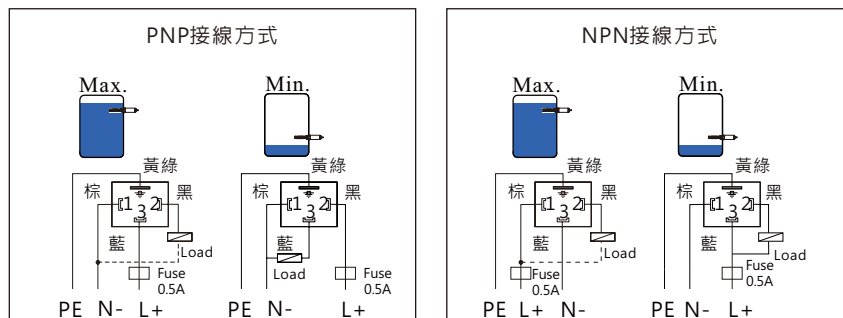
M12x4Pin接線圖
