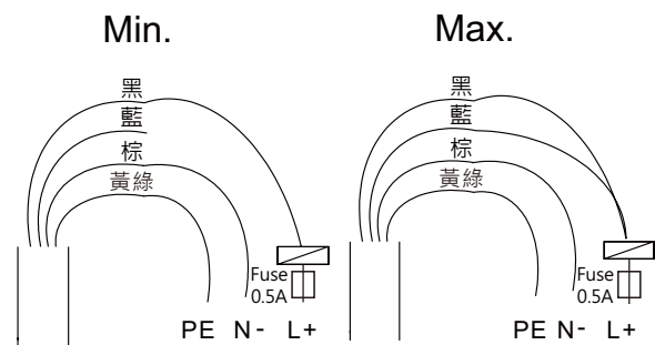
M12x4Pin、Cable 接線圖
