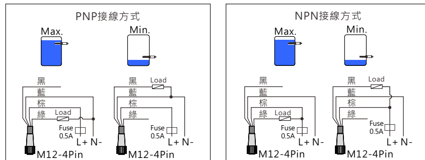
圖(二) PNP/NPN輸出之接線方式
