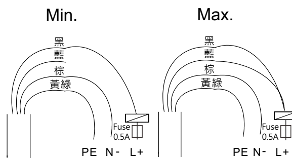
M12x4Pin、Cable 接線圖
