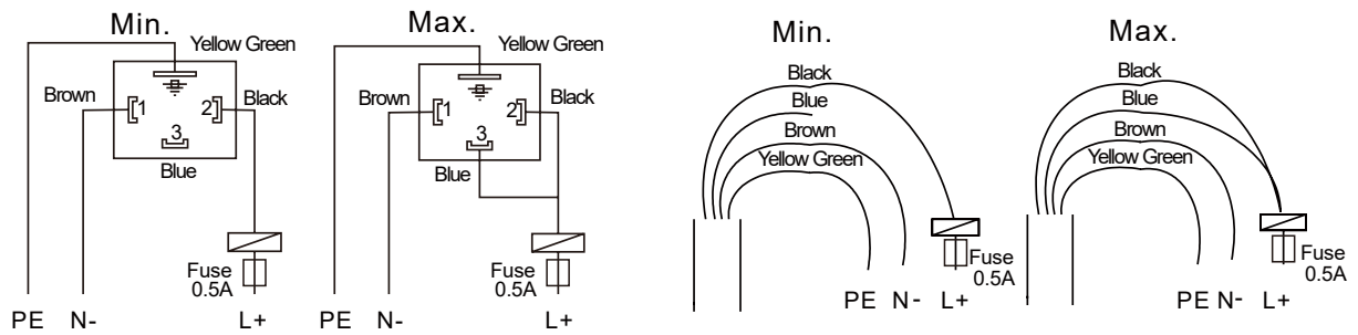
DIN Wiring Diagram
