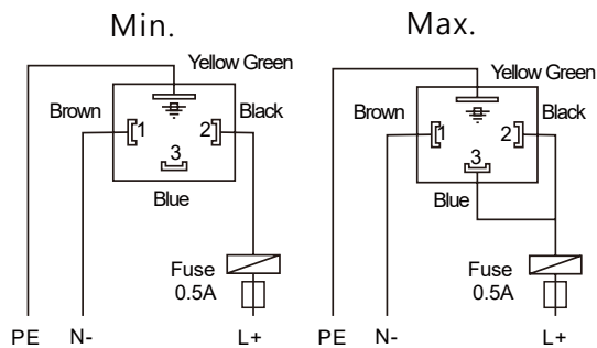
DIN Wiring Diagram
