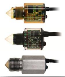
光電開關
