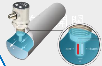
漏液偵測感測器
