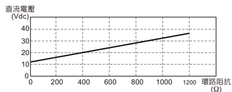
(圖四)最小驅動電壓與環路阻抗
