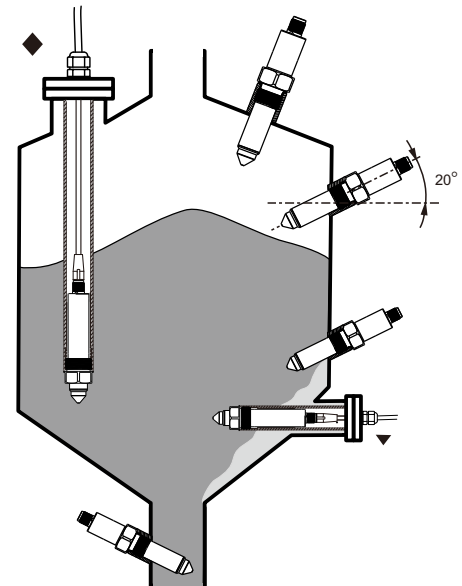
桶槽示例
