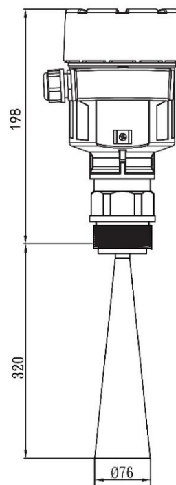
JFR484 外觀尺寸
