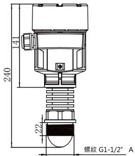
JFR481 外觀尺寸
