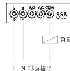
接法1(圖1)
