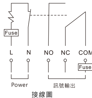
接線圖
