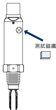
圖(三) 磁性測試示意圖
