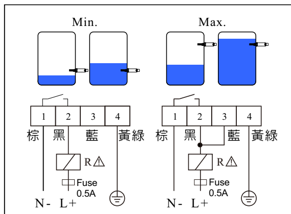
圖(一) 兩線式電源接線
