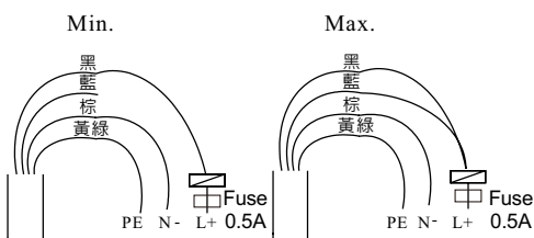
M12x1、Cable 接線圖
