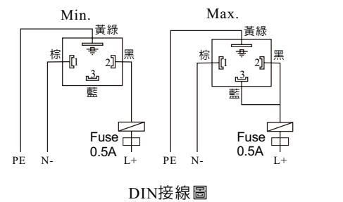
DIN接線圖
