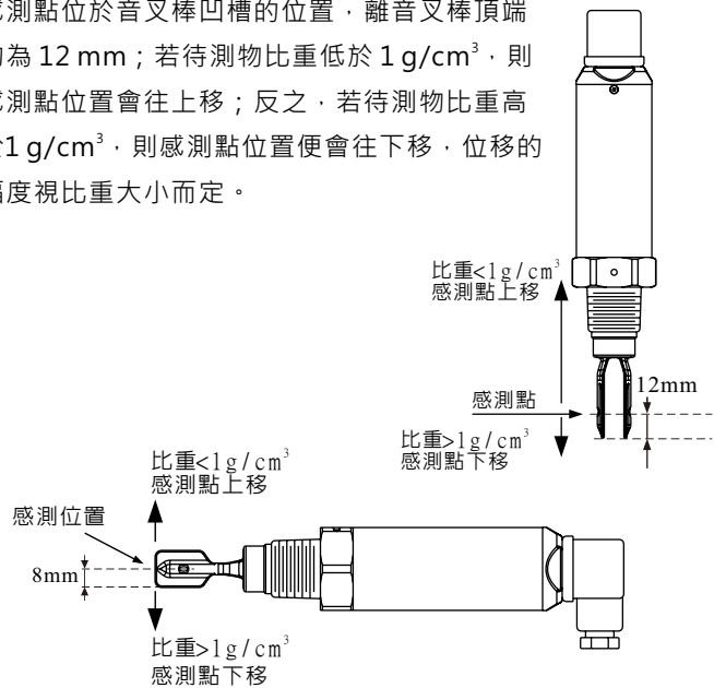
圖(二) 振動棒感測位置
