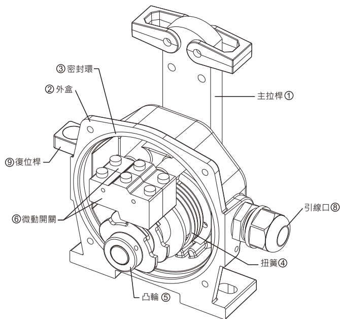
(圖1)構造圖
