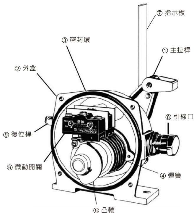
圖1 構造圖
