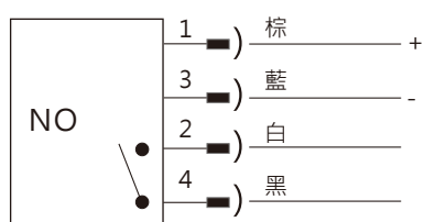
圖 9 SPC2 繼電器輸出型(NO)
