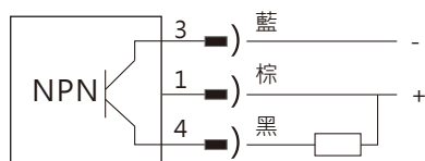
圖 6 SPX2 NPN 輸出型
