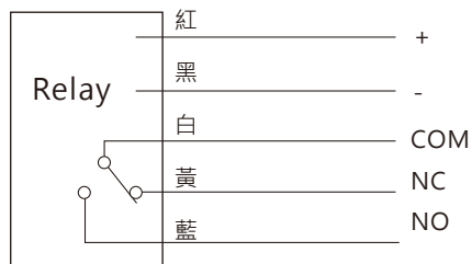
圖 8 SPX1 繼電器輸出型
