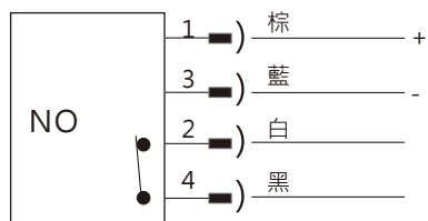
圖 10 SPX2 繼電器輸出型(NC)
