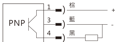
圖 7 SPX2 PNP 輸出型
