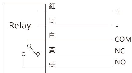
圖 8 SPX1 繼電器輸出型
