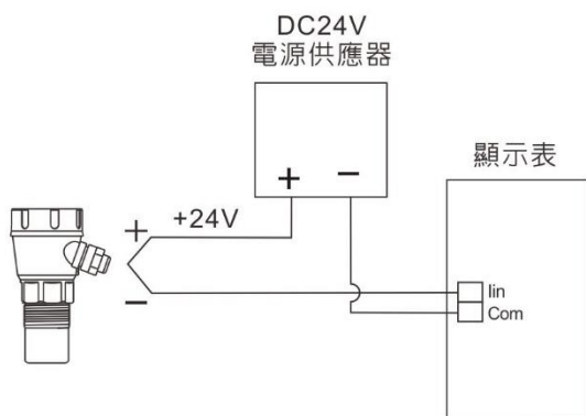
二線式 (外部供電)
