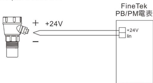
二線式 (盤面電錶供電)
